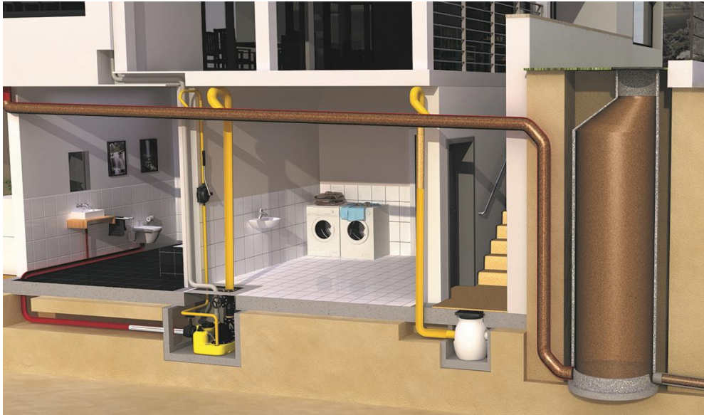
Bild 3: Die Hebeanlagen werden über Rückstauschleifen angeschlossen, die über die Rückstauenebene führen. So wird ein Rückstau vermieden.
